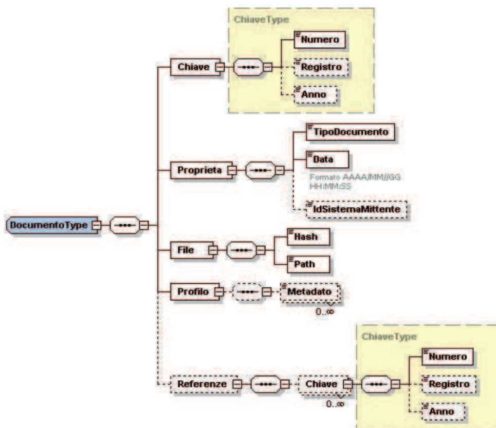
Figura 3 - Nodo documento
