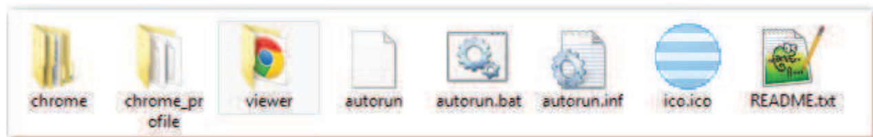
Figura 4 - Struttura volumi
