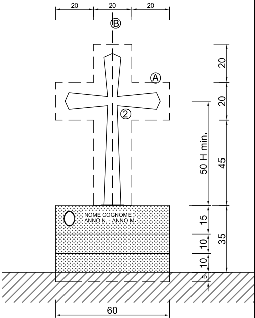
VISTA FRONTALE
